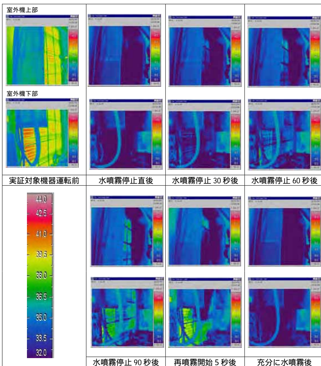
図 4 - 3 熱交換器フィン表面の温度変化
